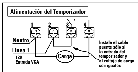
ET1105 configurado para SPST, carga de 120 V CA
