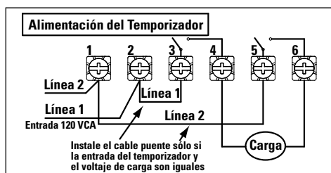
ET1125 configurado para carga DPST 240 V CA con cable puente ajustado en SIM
