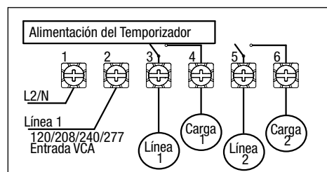
ET1125 configurado para 2 cargas SPST con cable puente ajustado en IND
