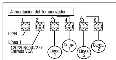
ET1125 configurado para cargas DPST con cable puente ajustado en SIM
