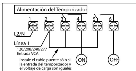
ET1125 configurado para carga SPST de pulso con cable puente ajustado en PUL
